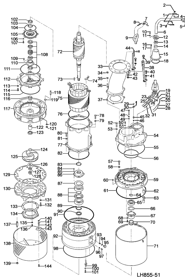
LH855-51
